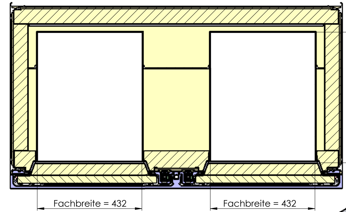
A-A (1:8)
